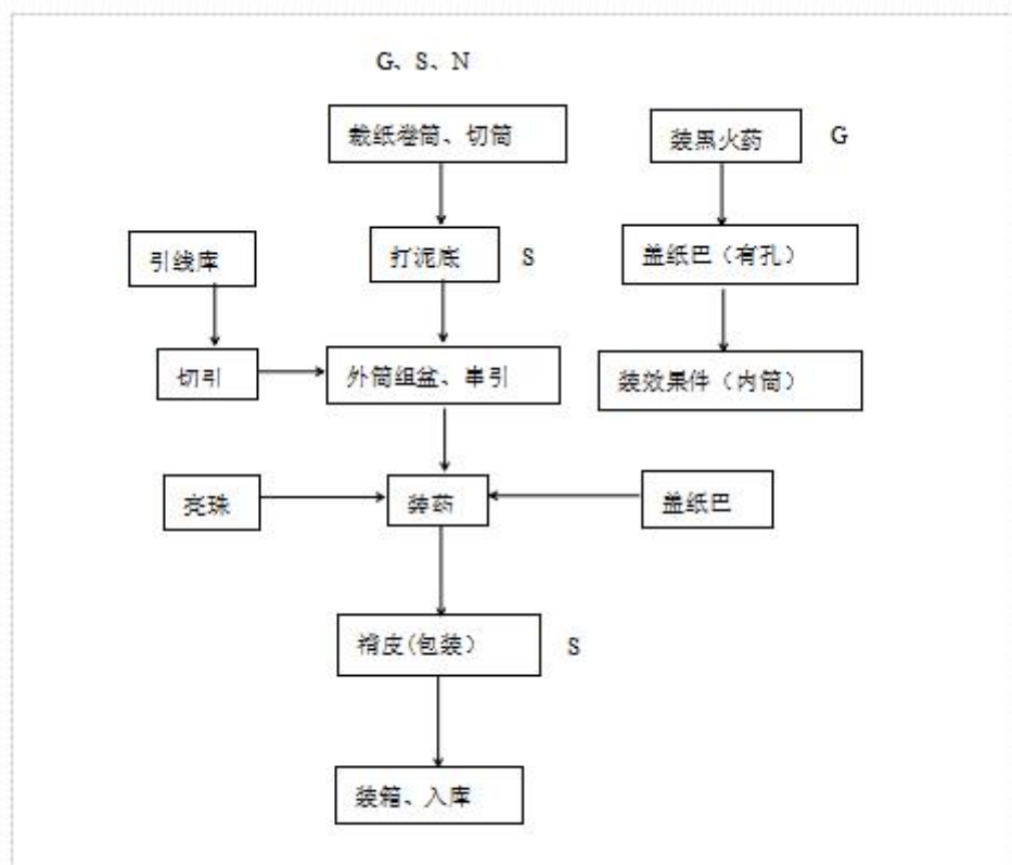
图1 组合类烟花生产工艺流程及产污节点图
